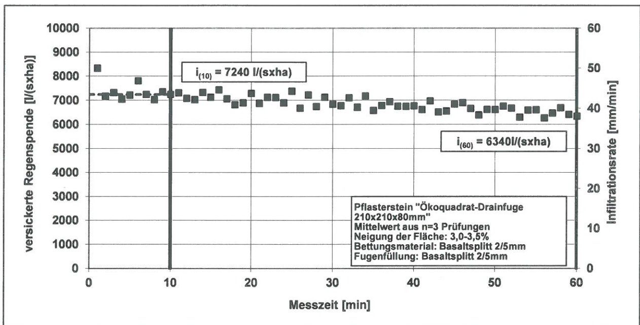
Abb. 3: Ergebnisse der Infiltrationsmessung
