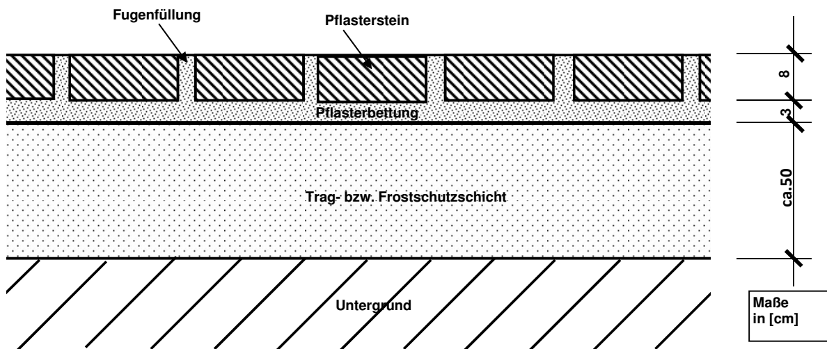
Abb. 1: Aufbau des Versickerungssystems (Prinzipskizze)
